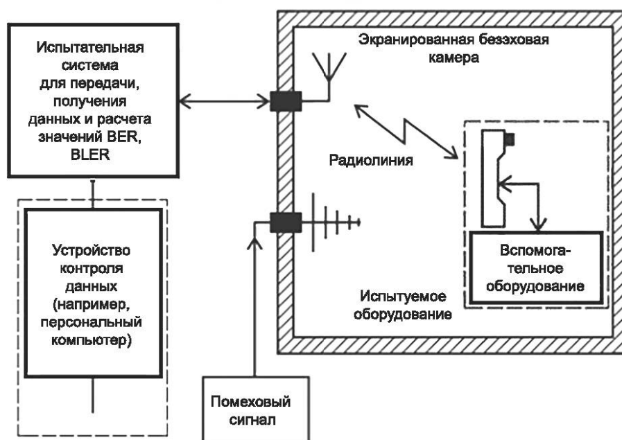
Рисунок С.2 — Схема испытаний при наличии вспомогательного оборудования обработки данных
